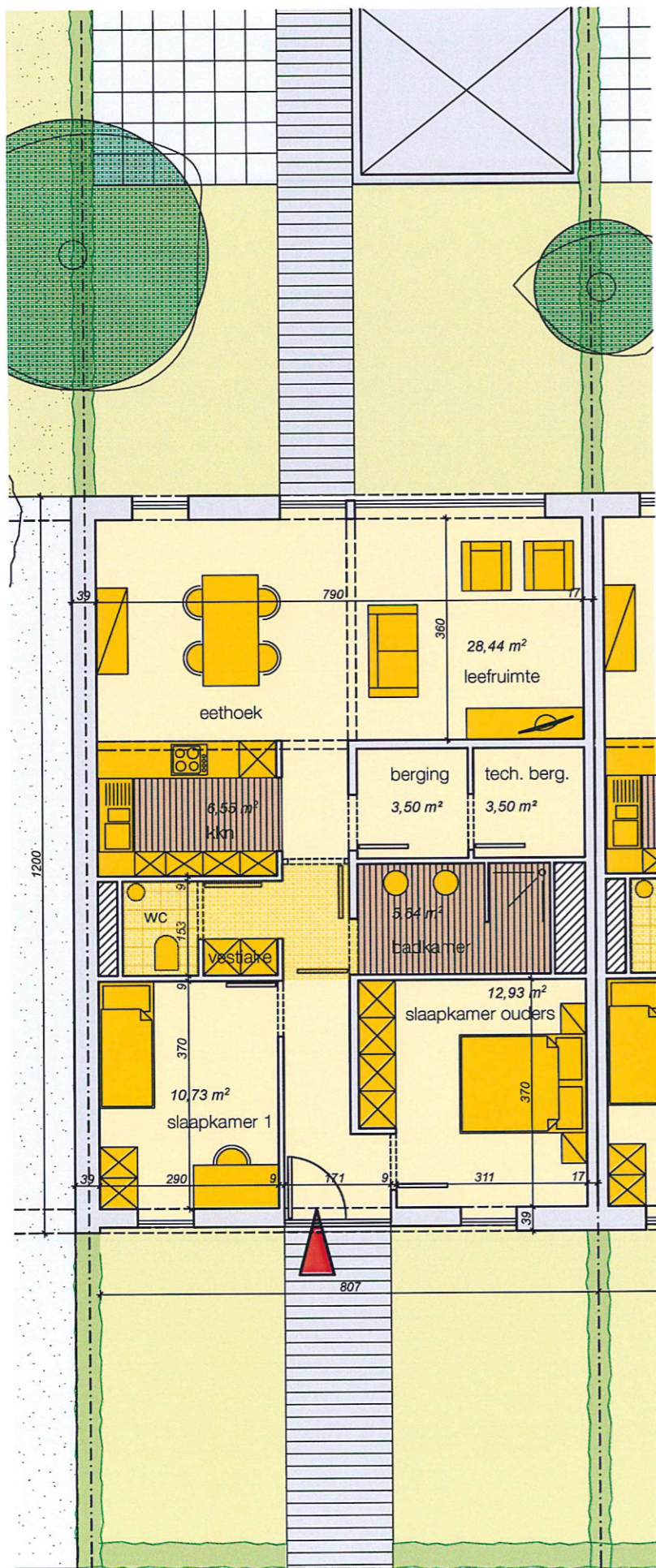
plan gelijkvloerse verdieping 1/100 appartementen lot 26
