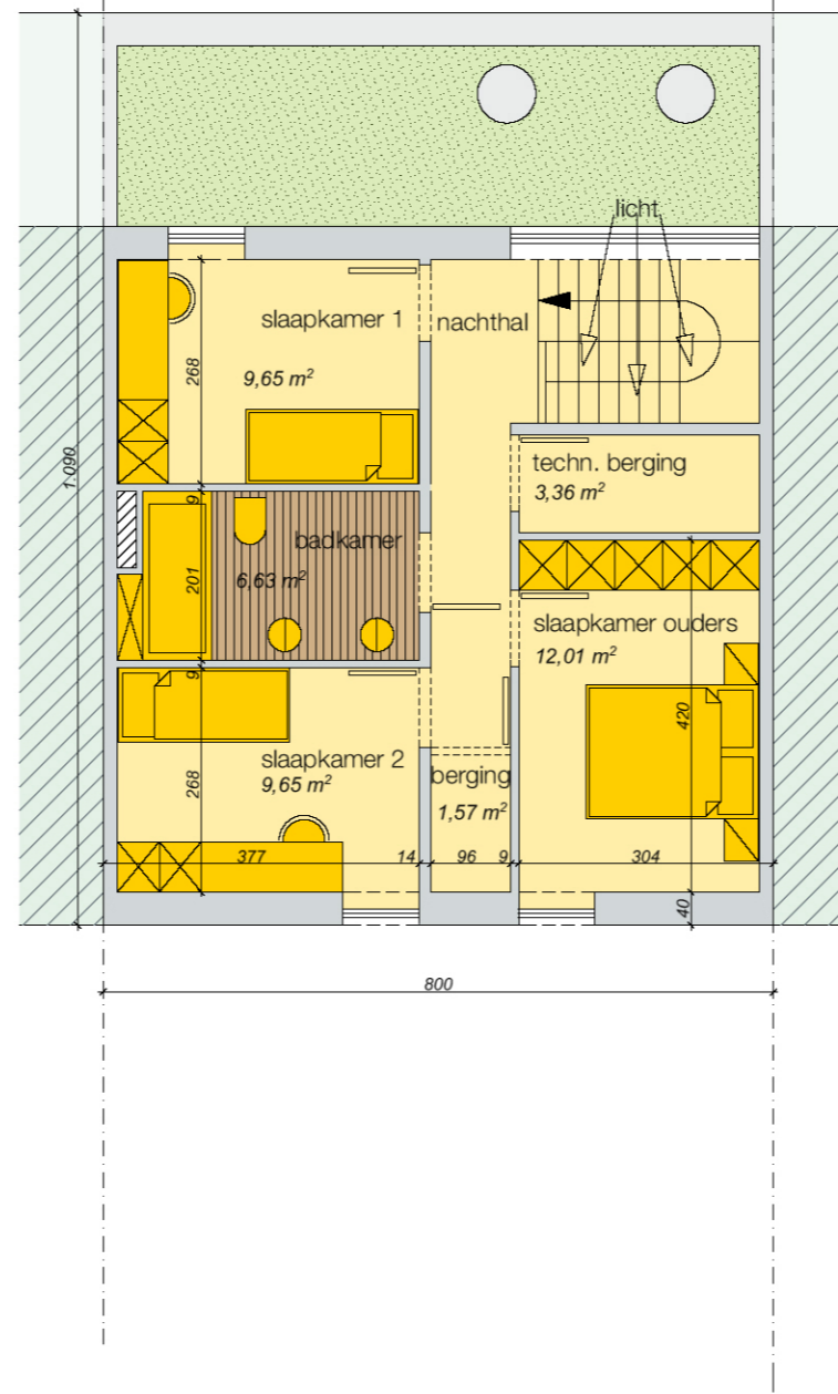
plan 1e verdieping 1/100
