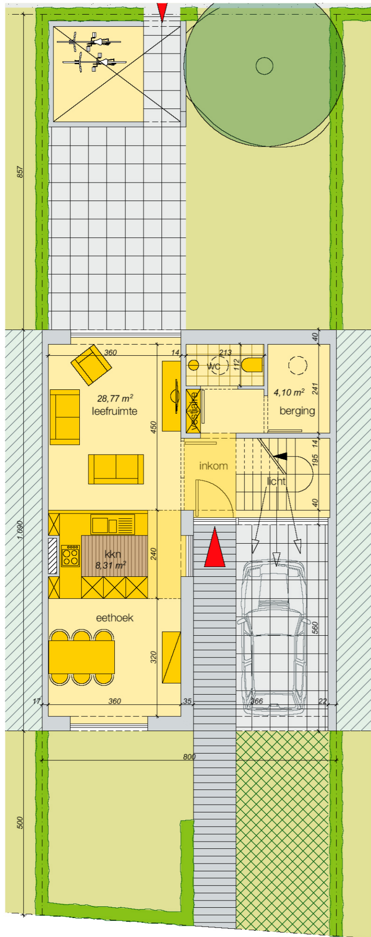
plan gelijkvloerse verdieping 1/100 rijwoning lot 40/ 3 slaapkamers 4 personen
