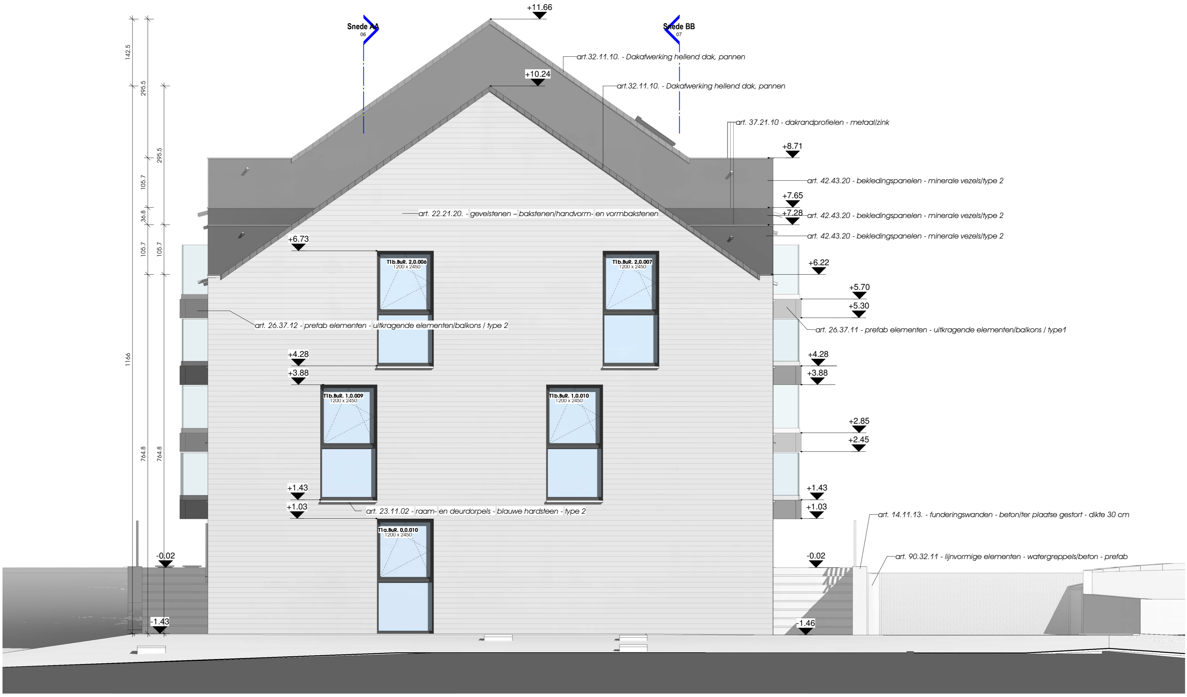
2 Zuidgevel 1 : 50
